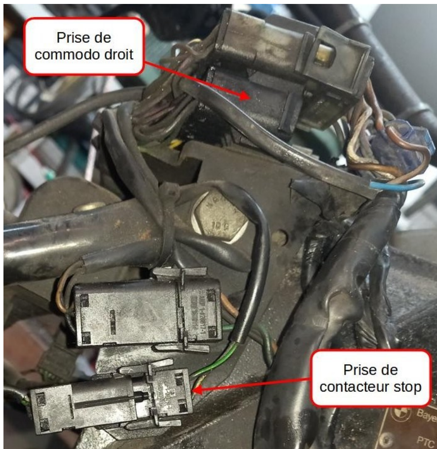
La prise du contacteur de stop avant fixée à droite de la partie avant du cadre
